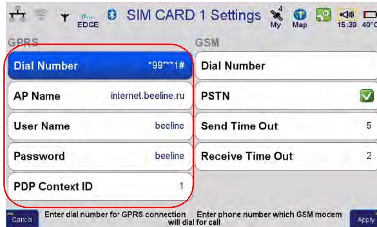
Figure 8. GPRS Parameters
